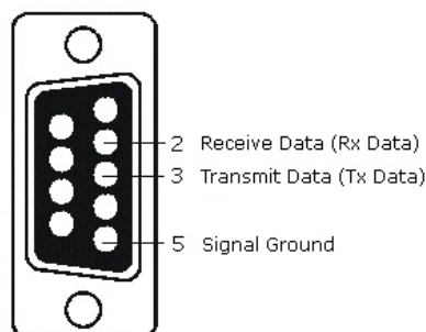
圖 A、DB-9 連接頭 PIN-OUT。
