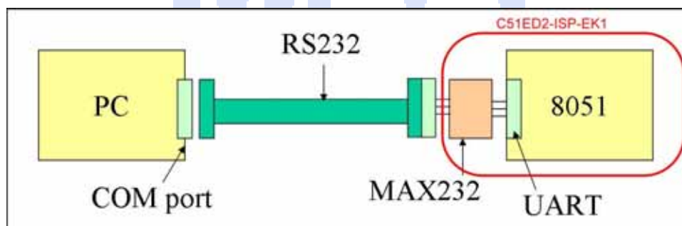
圖一、C51ED2-ISP-EK1 實驗板與個人電腦連接示意圖。
